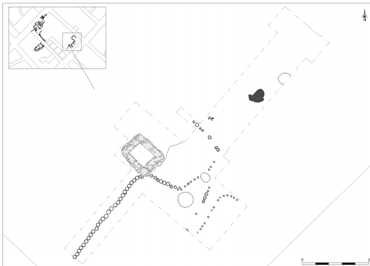
FIGURA 8. Planta de les restes documentades del centre terrisser. Font: Mario Granollers.
